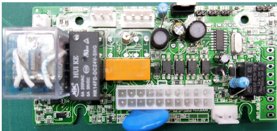
EPS-SIG 信号板布局图
