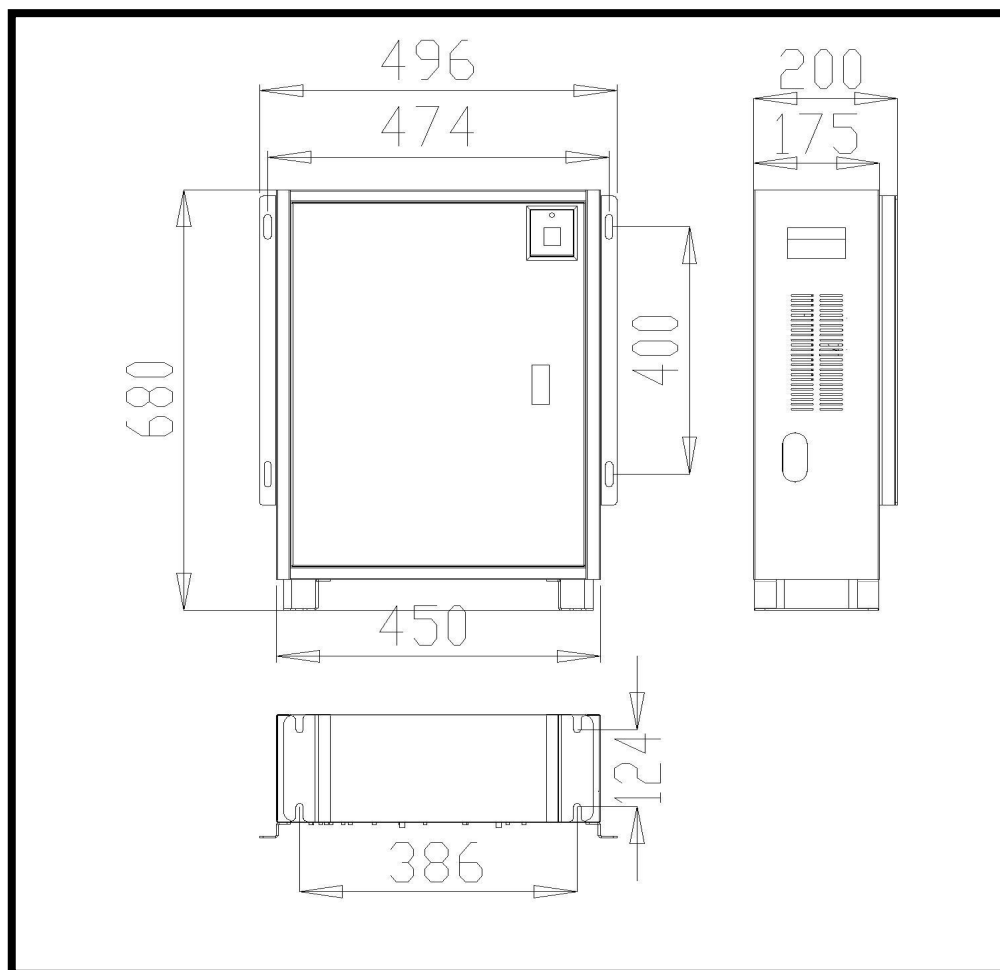
功率<30KW 装置安装尺寸图
