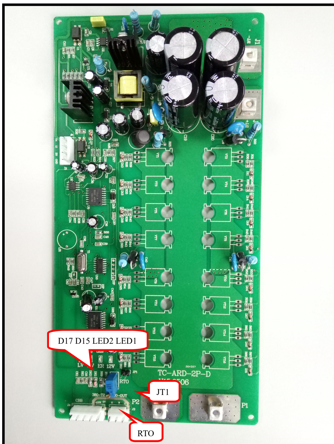
ARD-D 逆变板布局图
