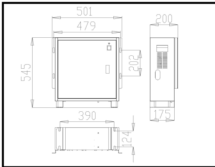
功率<15KW 装置安装尺寸图
